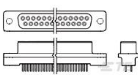
TE 产品编号207841-3 09 RCPT SP/AP INSRT
