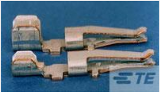
TE 产品编号556135-2 CONT,AMPINNERGY WTW,LS PC,14-18
