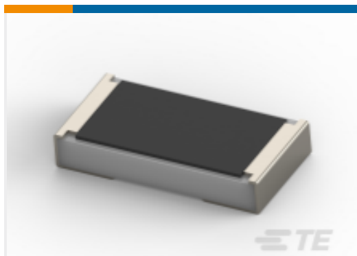
TE 产品编号2176231-9 SMD 功率电阻器：3 瓦特，1% Tol
