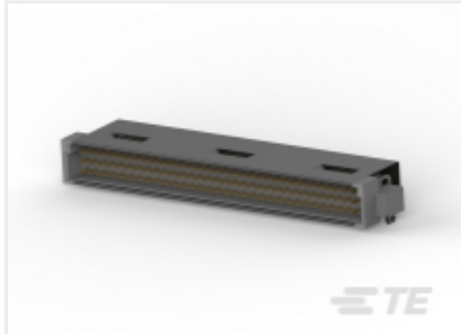
TE 产品编号 5536148-5 ASSY,PIN,ENH.TYPE C,EUROCARD,L-FREE,5ROW
