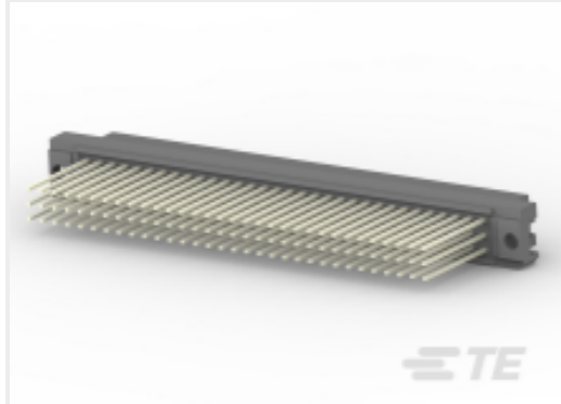
TE 产品编号 1-148059-5 096 EURO TYP C RECP 17MM ASSY
