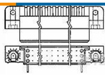
TE 产品编号533268-6 HDI RECP ASSY 3 ROW 135 POS
