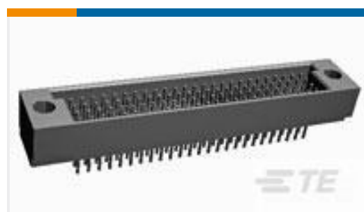
TE 产品编号 5532448-9 ASSY,PIN,VERTICAL,HDI,LEAD-FRE
