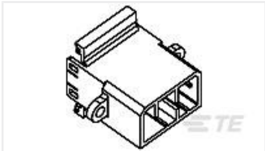
TE 产品编号1-174937-1 070 MLC W-W CAP HSG 8P F/A
