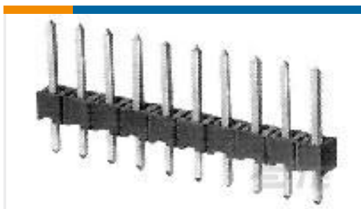
TE 产品编号826630-2 2P AMPMODU II STIFT LEI
