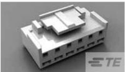
TE 产品编号1-1123722-0 3.96 EP PLUG HSG 10P(NATURAL)
