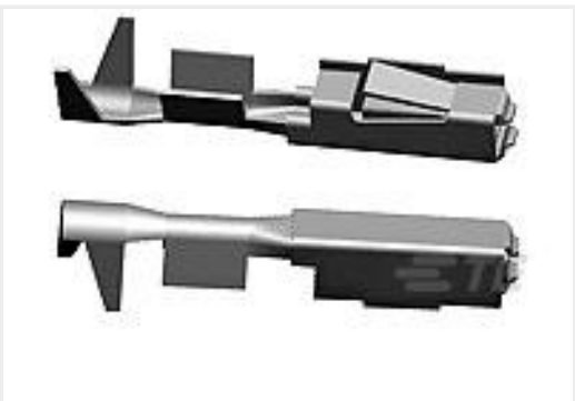
TE 产品编号5-968221-6 MQS0,63 Ag rec CB unseal. 0,5-0,75
