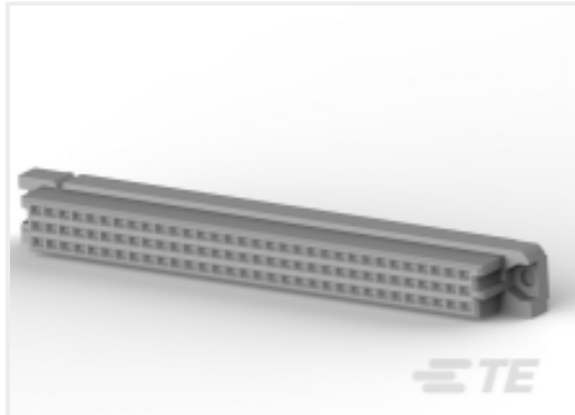
TE 产品编号 5535032-5 ASSY,RECEPTACLE,EUROCARD,TYPE C,LEAD-FRE
