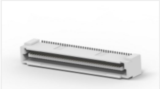
TE 产品编号 CAT-313-PCB80 自由高度插头连接器：板对板, 垂直, 80, 0.8mm
