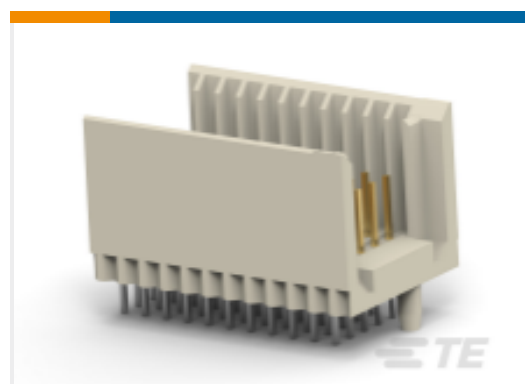
TE 产品编号5646346-1 硬公制公连接器：传统背板，夹层，2mm
