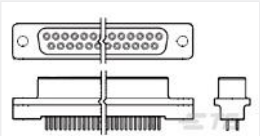
TE 产品编号5745078-6 HD-20 RCPT 25P VERT FFSCRLK
