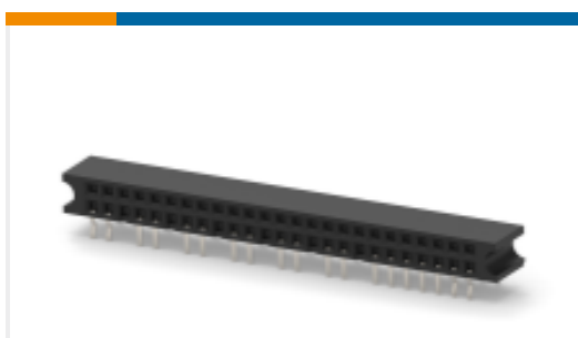
TE 产品编号 5-535525-1 MODII RECP ASSY 50 POS
