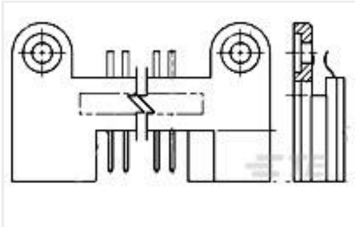
TE 产品编号1-530785-2 BOX PIN HDR ASSY 50 PS 075 CL
