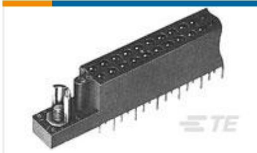
TE 产品编号531813-2 BOX RECP 150 POS STAG
