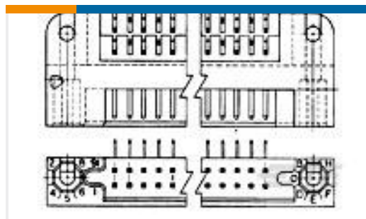
TE 产品编号1-531720-3 2 ROW BOX PIN 150 POS R/A
