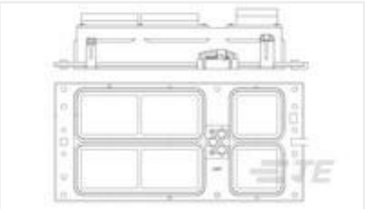
TE 产品编号YDTS20F19-35ABV001 RECP ASSY
