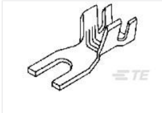
TE 产品编号61855-1 SPADE 10-6 AWG TPBR
