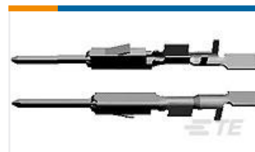
TE 产品编号1355719-2 MQS0,63 Au tab LL unseal. 0,08-0,22
