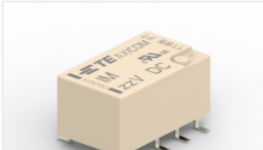
TE 产品编号1462047-1 IM48IGR=IM RELAY 100mW 2.4V BIS
