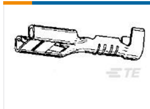
TE 产品编号282178-1 FF 250 REC 0.3-0.8MM2 BR
