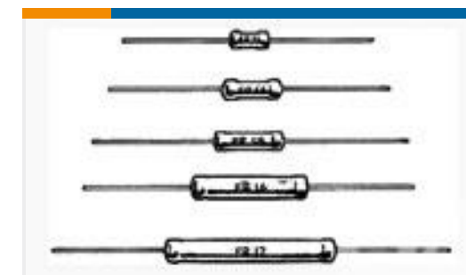
TE 产品编号4-1623750-9 ER58 R47 5% AMMO
