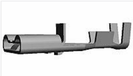
TE 产品编号170327-1 250 PL MKII REC. 22-18AWG PTBR
