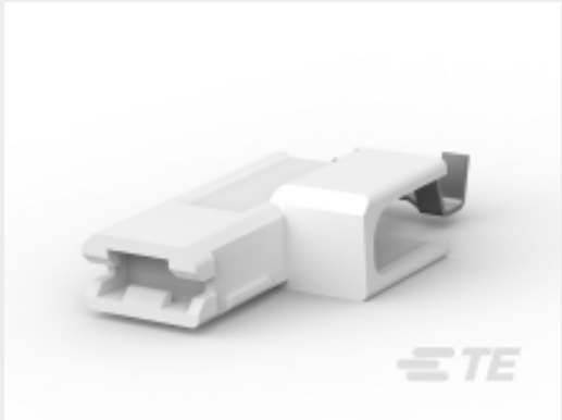
TE 产品编号CAT-UL8-187 ULTRA POD：旗形，母端组件，镀锡，0.187 英寸
