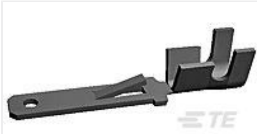
TE 产品编号60294-1 FF 250 TAB 22-18AWG BR
