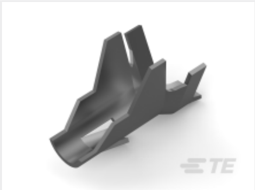
TE 产品编号343445-2 AMP-IN MINI (SPECIAL) 18.5-14 AWG
