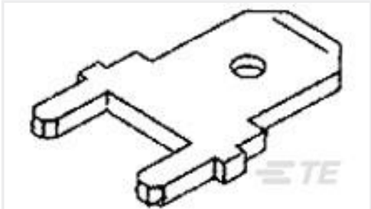
TE 产品编号63603-1 187 FASTON TAB TPBR
