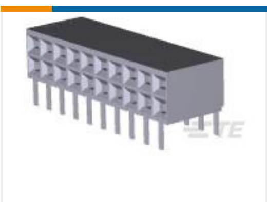
TE 产品编号5535512-2 20 MODII HORZ DR CE
