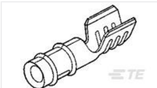
TE 产品编号640024-1 058 PIN REC 010TP
