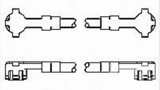
TE 产品编号1064533-1 9960 1305 24
