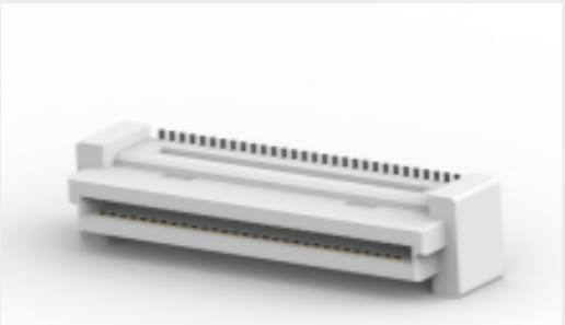
TE 产品编号 CAT-313-RCB60 自由高度插座连接器：板对板，垂直，60，0.8mm
