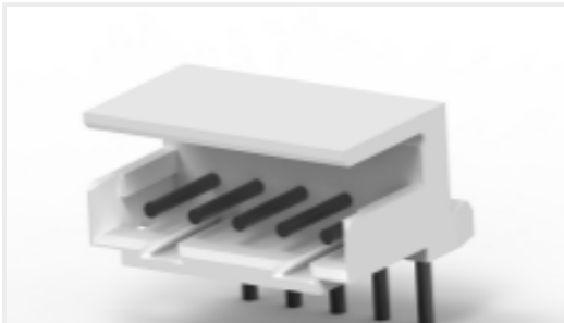
TE 产品编号CAT-3983174-PHBXHK CT 2mm 柱公端组件 Box H 扭结
