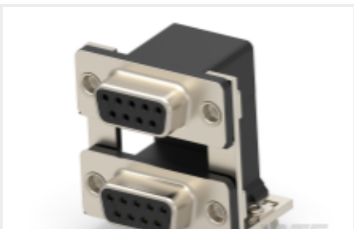
TE 产品编号2454917-1 D-SUB ,9 POS RCPT OVER 9 POS RCPT
