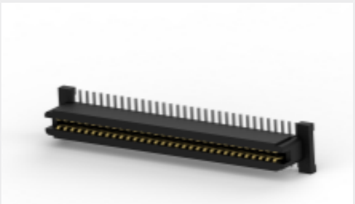
TE 产品编号 CAT-314-RCB64 自由高度插座连接器：板对板，垂直，64，1mm
