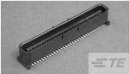
TE 产品编号 2007042-1 1FHR,64,50A/P,S,C,R08,09,10
