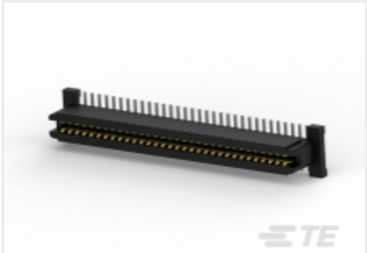
TE 产品编号 CAT-314-RCB64 自由高度插座连接器：板对板，垂直，64，1mm
