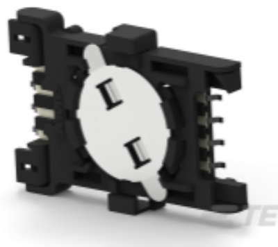
TE 产品编号 5145299-2 SIM/SAM RECPT,6 POS,SMT
