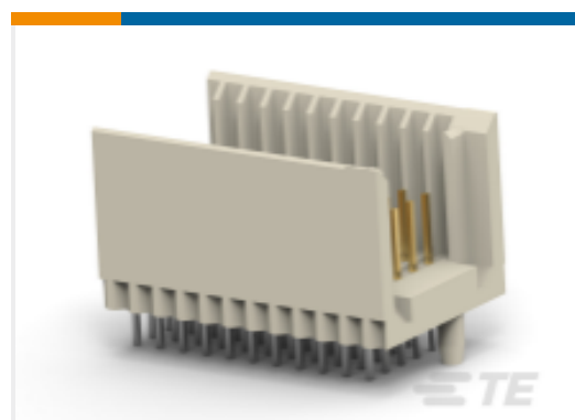
TE 产品编号5120638-1 硬公制公连接器：传统背板，夹层，2mm
