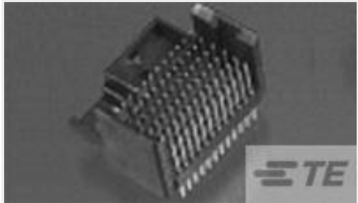
TE 产品编号 5120642-1 2MM HM HDR ASY,12 ROW 072 R H
