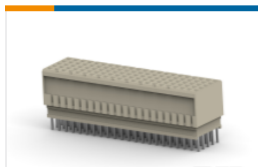
TE 产品编号5120640-1 硬公制背板母端连接器：夹层，2mm
