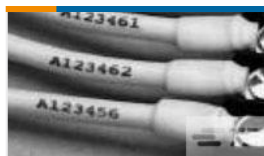
TE 产品编号 5053182032 RNF-100-3/8-9-STK
