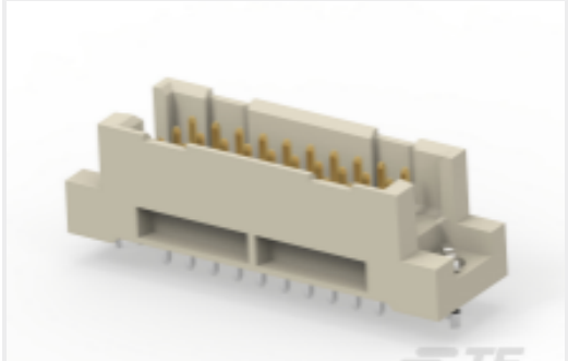
TE 产品编号374857-E STVR/3 30 MI ABC VV 4-00 GA06 2,5 * 247
