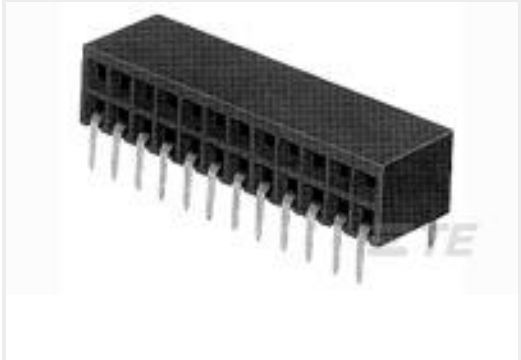
TE 产品编号216604-7 2X 7P HV190FEDERLEI
