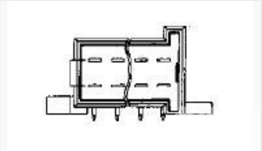
TE 产品编号828801-5 2X 7P MESSERLEI 3,0
