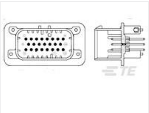
TE 产品编号 776228-1 23POS,PIN DIA 1.3,HDR ASSY, 180DEG,COD 1
