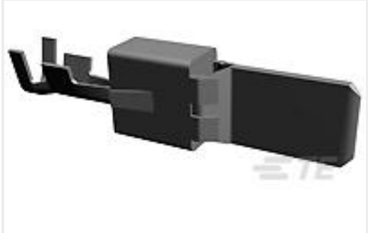
TE 产品编号963768-1 TAB 9.5x1.2 CONTACT CS SRC Sn
