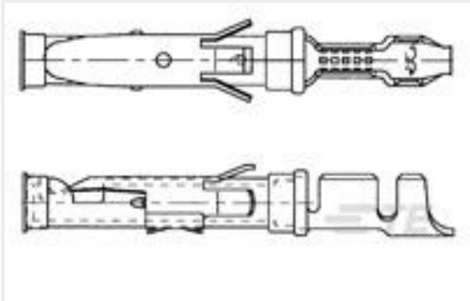
TE 产品编号 164840-2 062 M SRS.SOCKET 3+
