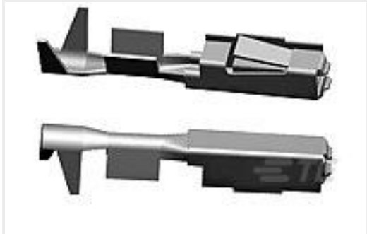
TE 产品编号 5-963715-6 MQS0,63 Ag rec LL unseal. 0,5-0,75
