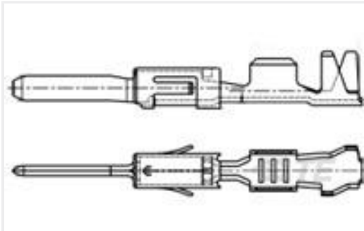
TE 产品编号 963904-1 TAB A 1.6x0.6 CONTACT CS SWS Sn
