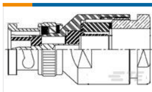
TE 产品编号1-1478404-0 BNC Str Plg PS 75Ohm Silver RG59B /U, 62A
