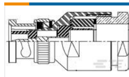
TE 产品编号1-1478403-0 BNC Str Plg PS 75Ohm Silver RG179B /U, 18
