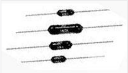
TE 产品编号1879656-7 H8 178K 0.5% 100PPM
