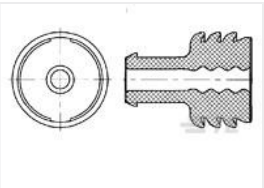
TE 产品编号967653-1 MPQ BLINDSTOPFEN6,4
