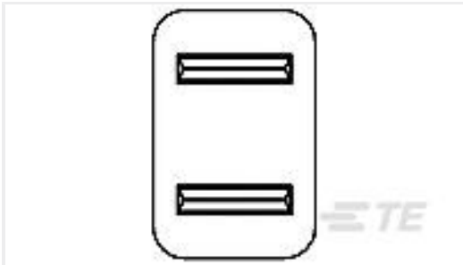
TE 产品编号 963203-1 SEALING F/2P 5.8MM TAB HSG
